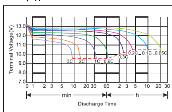
Разрядный ток 25°C
