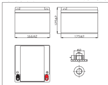
Клеммы T0
